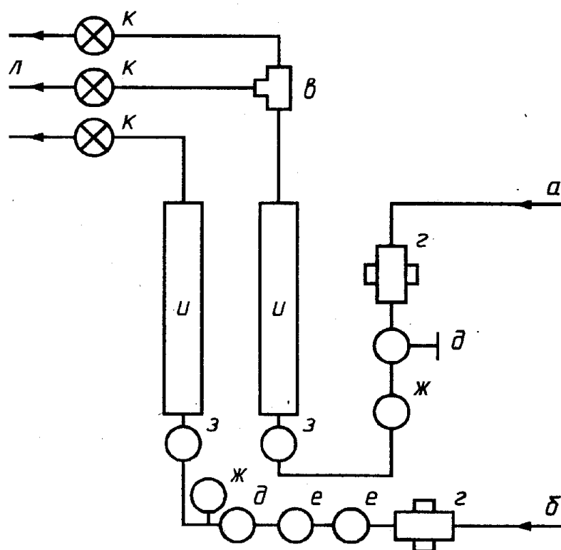
Рисунок 4а — Сдвоенная горелка
