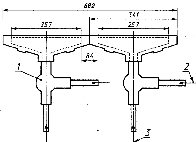
Рисунок 4а — Сдвоенная горелка
