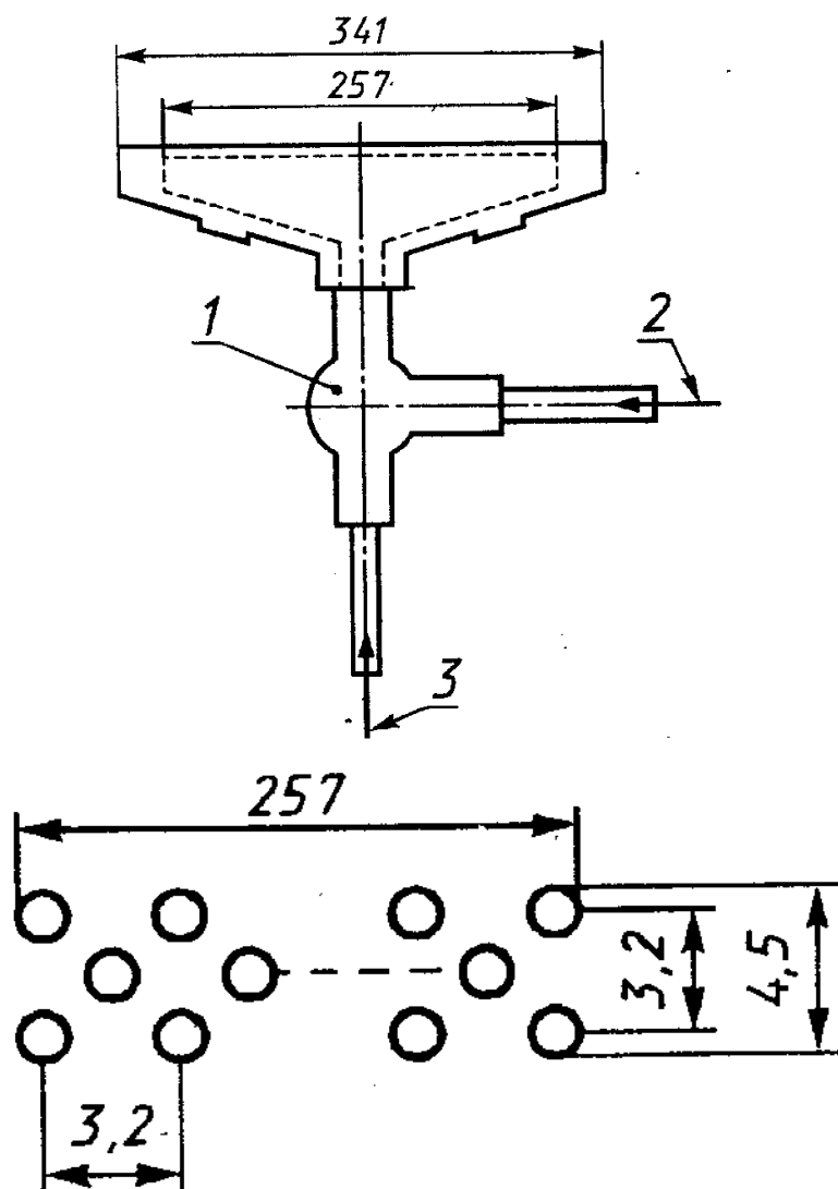
1 — смеситель Вентури для воздуха и газа; 2 — вход пропана; 3 — вход сжатого воздуха Рисунок 4 — Горелка
