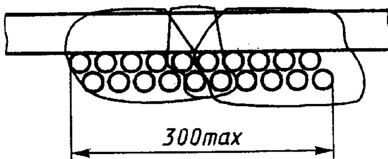
Рисунок 3г — Кабели небольшого диаметра, закрепленные на передней стороне стандартной лестницы (сформированные в пучки, кодовое обозначение A(F) )
