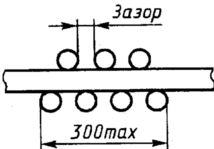
Рисунок 3б — Несоприкасающиеся кабели, закрепленные на передней стороне широкой лестницы ( A(F) > 35 \text{ мм}^2 )
