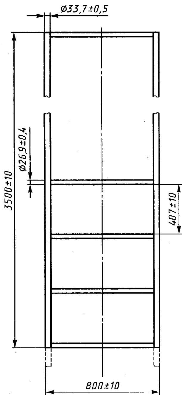
Рисунок 2а — Широкая трубчатая лестница для испытания кабеля. Число перекладин — 9
