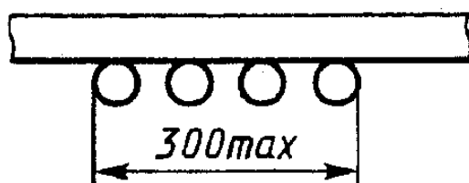
Рисунок 3а — Несоприкасающиеся кабели, закрепленные на передней стороне стандартной лестницы
