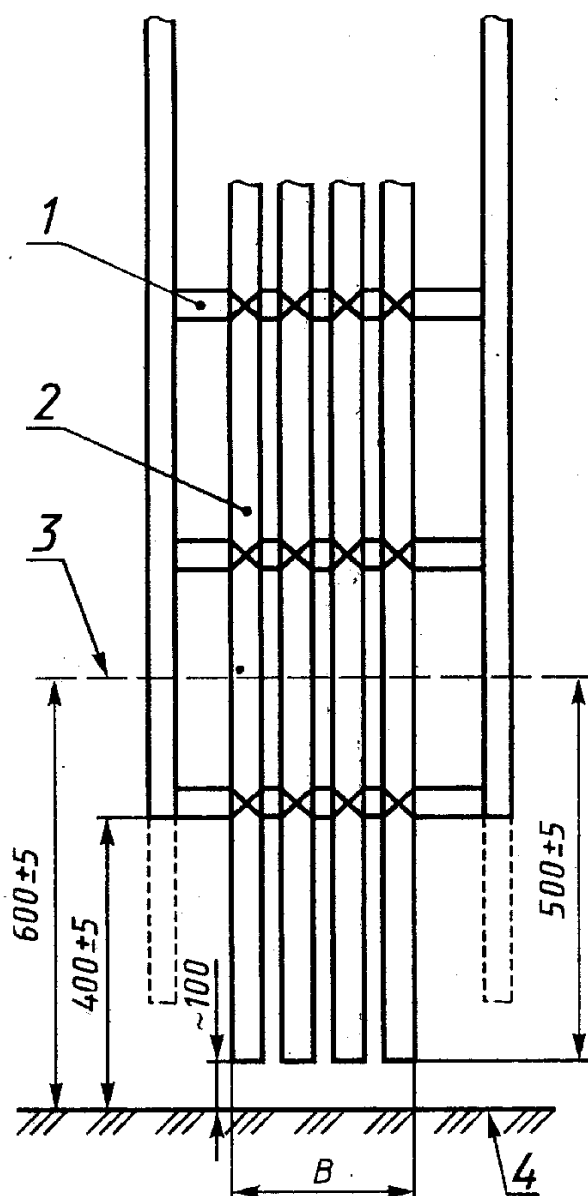
1 — круглые стальные перекладины; 2 — крепление металлической проволокой; 3 — центральная линия горелки; 4 — пол; B — максимальная ширина образца
